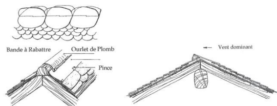
« Faîtage en lignolet, faîtage en plomb » et « Faîtage avec solin »
